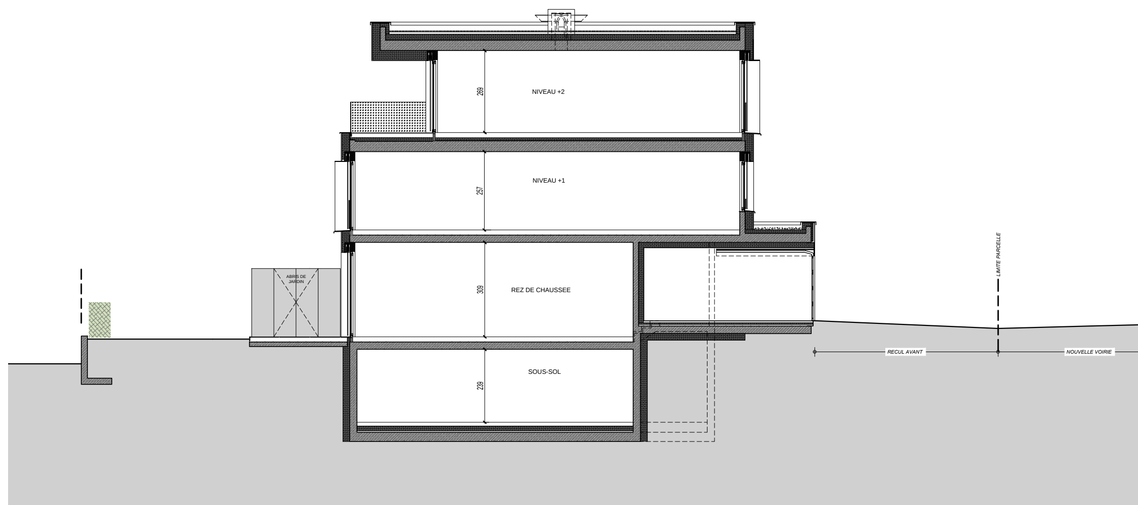
COUPE 1/125
