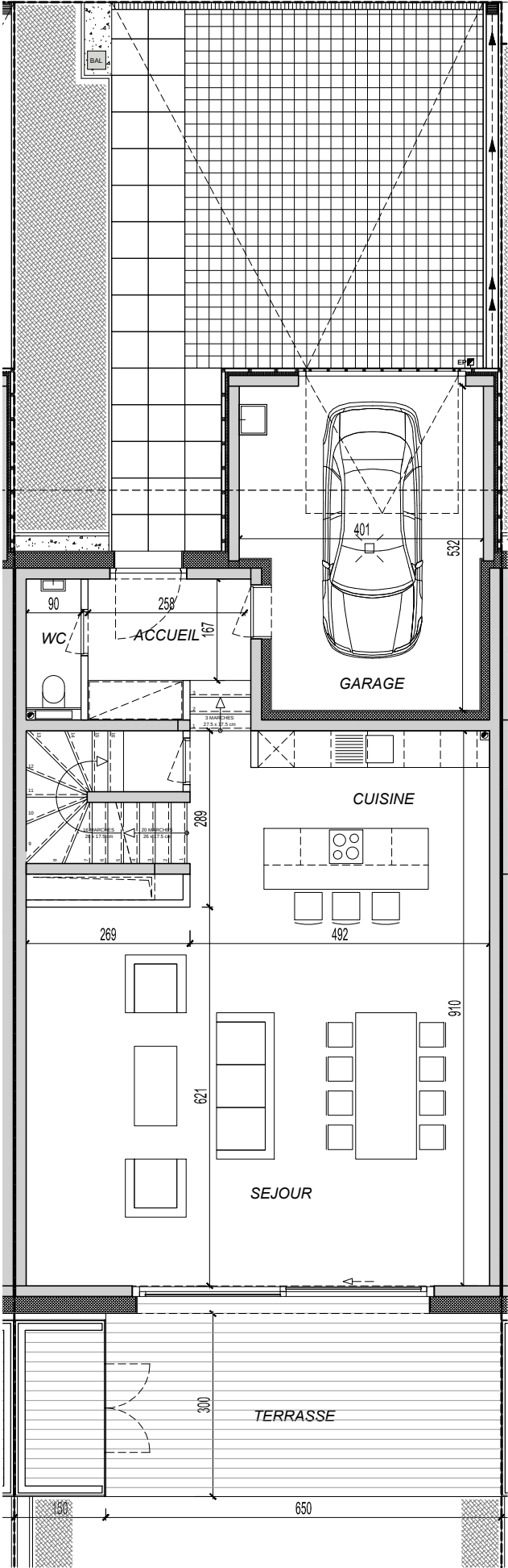
REZ-DE-CHAUSSEE 1/100
