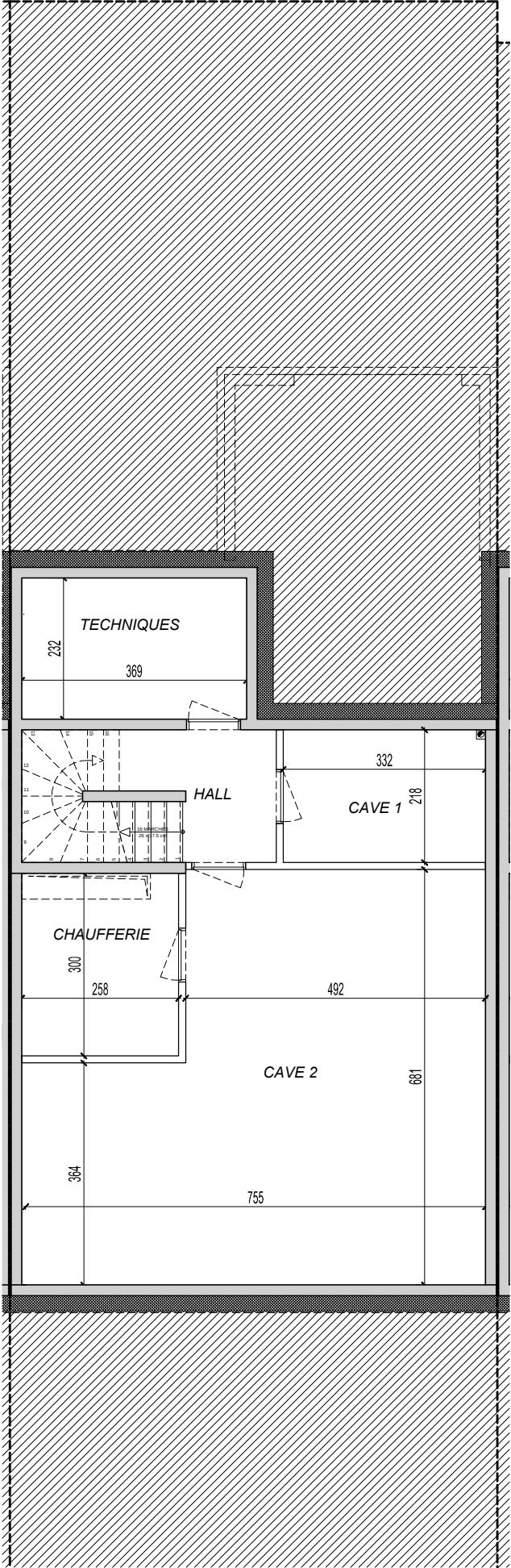
SOUS-SOL 1/100
