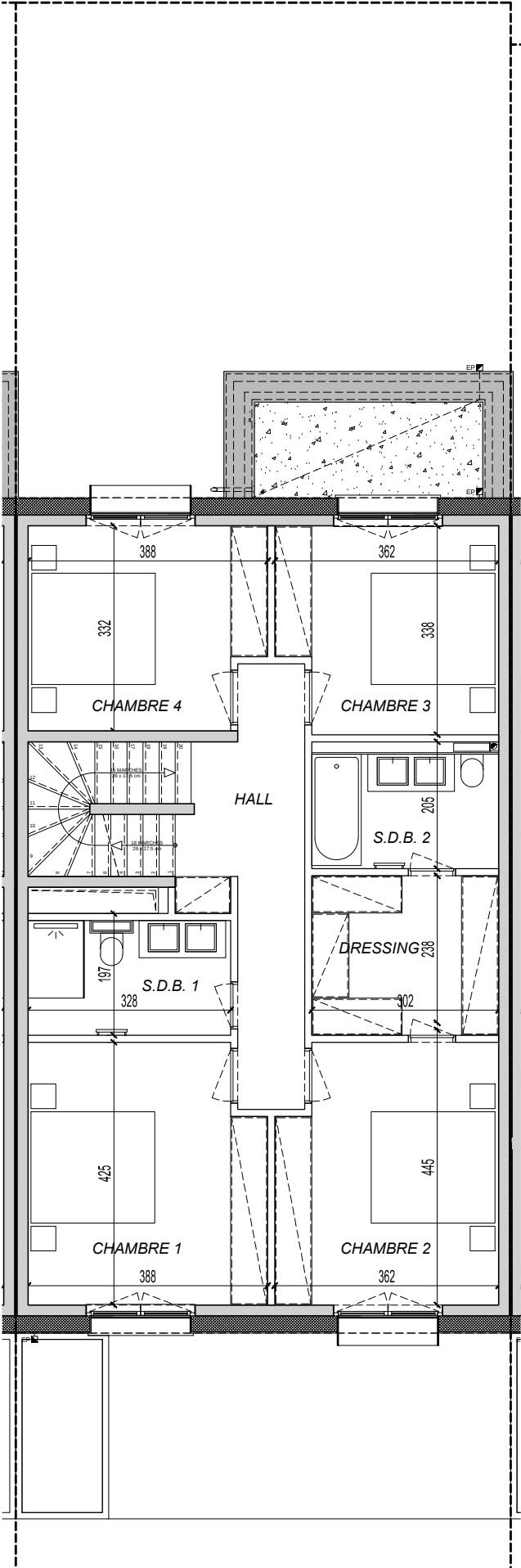
ETAGE 1/100
